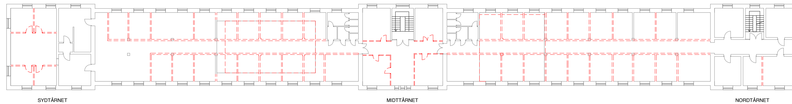
2 Plan 02 - riveplan 1 : 200
