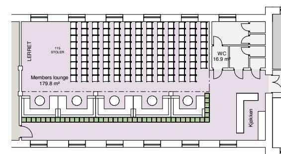
3 Members lounge ved forelesning 1 : 200
