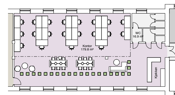
4 Members lounge som kontor 1 : 200
